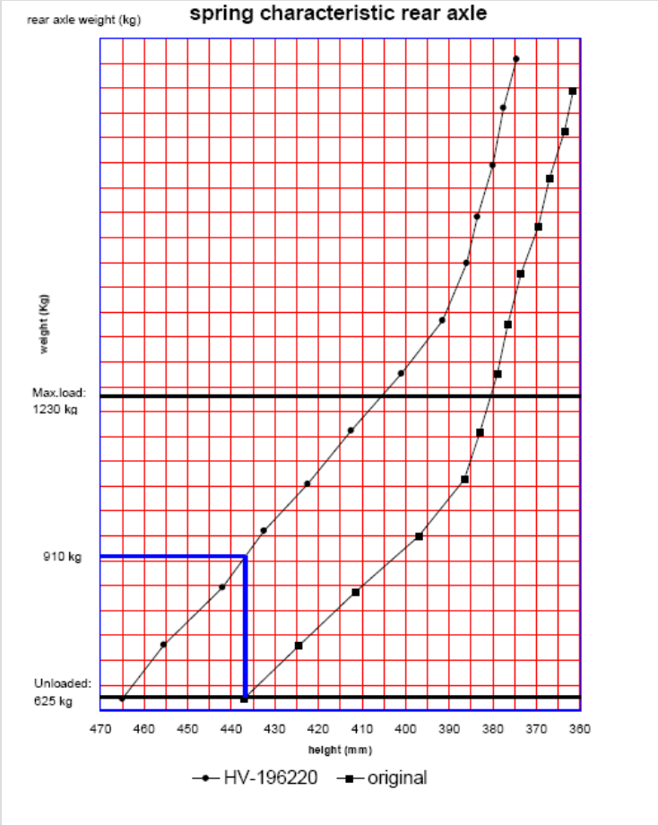
VW Caddy 0-system
