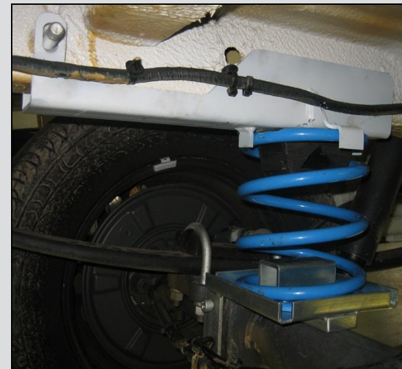
Mercedes Sprinter / VW Crafter 0-system
