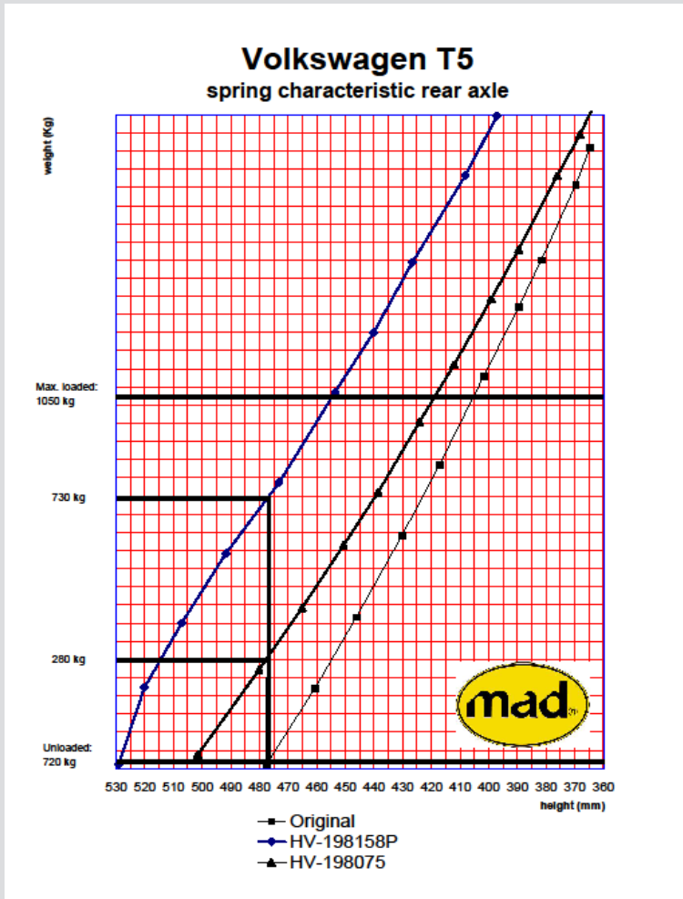
/ VW T 5/6 -system 8 system min. Load 600 KG
