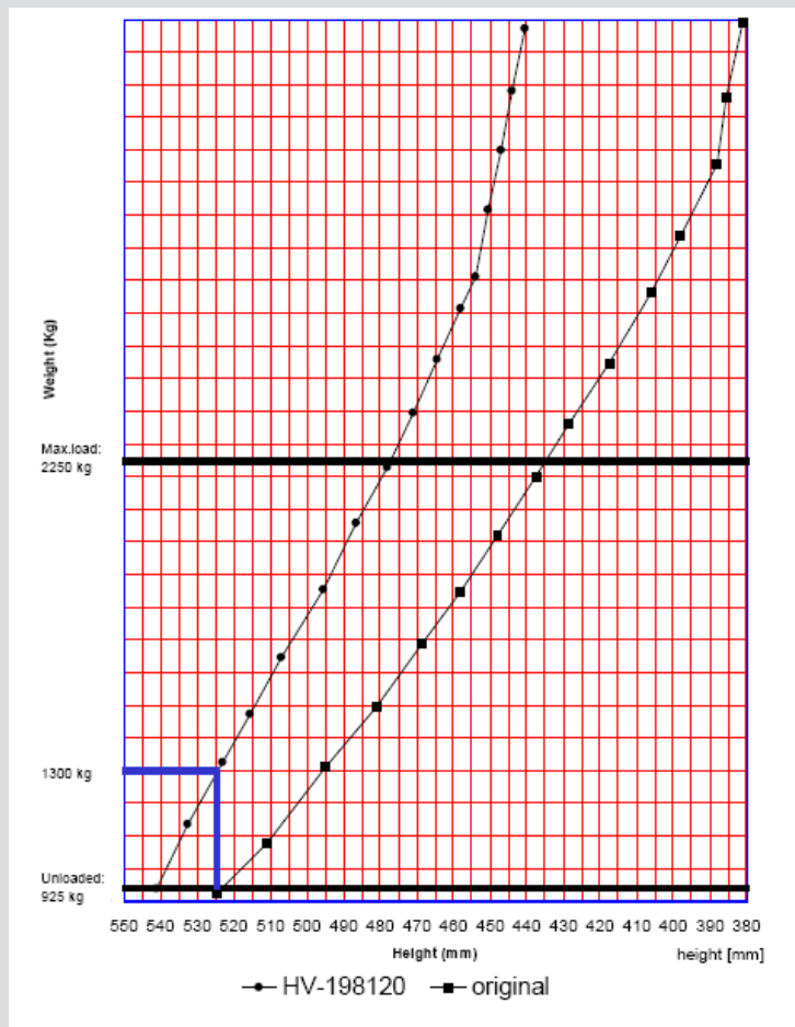
Mercedes Sprinter / VW Crafter 0-system
